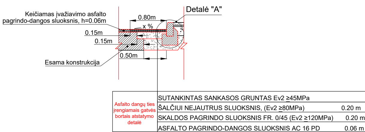
ASFALTO DANGŲ ATSTATYMO DETALĖ (šalutinėse gatvėse)
