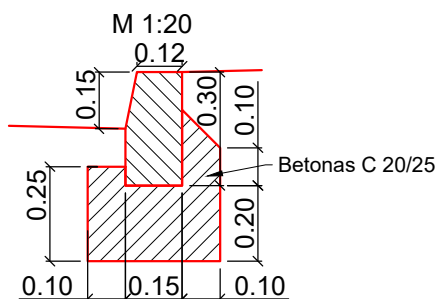
Detalė "A" Gatvės bortas 100x30x15
