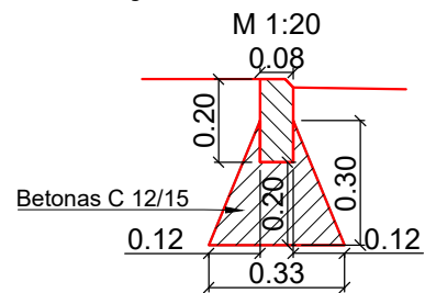
Detalė "B" Vejos bortas 100x20x8
